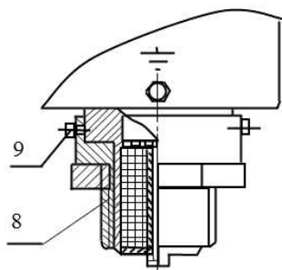
8 - штуцер; 9 - винт.
